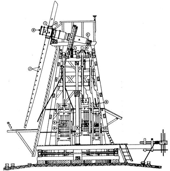
Doorsneden van de 'Zaanse' paltrok.
